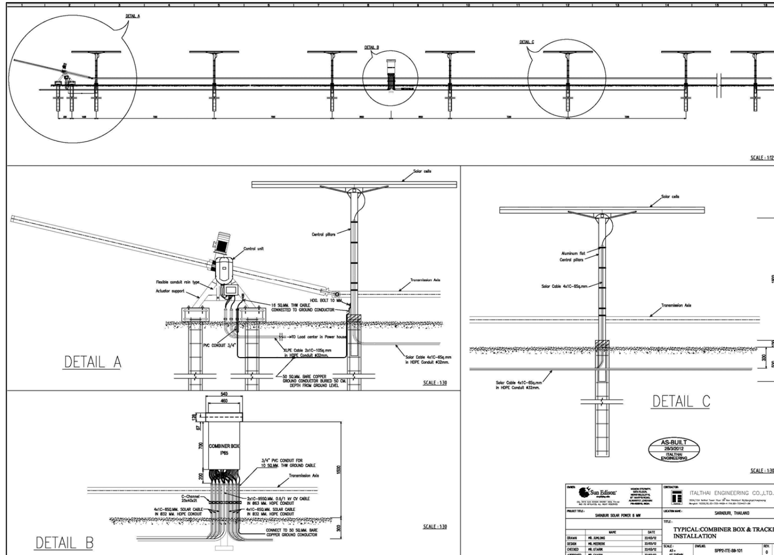
รูปที่ 2.2 โครงสร้างติดตั้งแผงเซลล์แสงอาทิตย์และเครื่องปรับองศาแบบแกนเดียว
